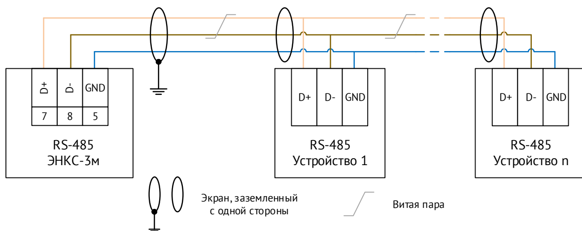
Рисунок 7.2. Подключение устройств по RS-485
