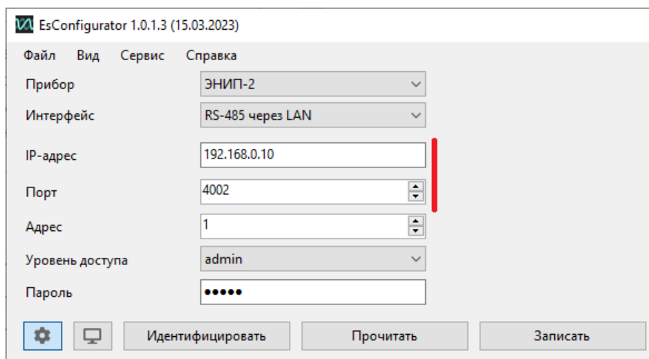
Рисунок 5.8. Пример настройки подключения к ЭНИП-2 с использованием «сквозного канала»
