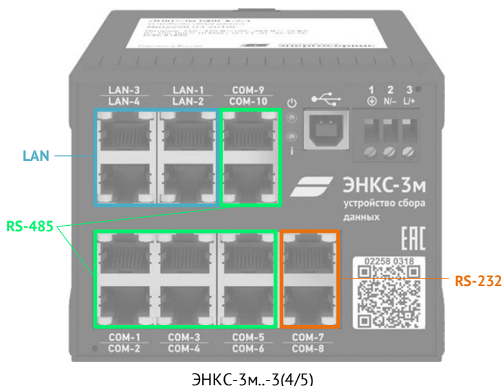
Рисунок 2.2. Соответствие интерфейсов ЭНКС-3м (hw 5)
